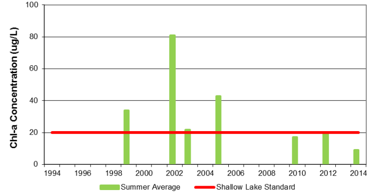
Lower Twin Lake Chlorophyll-a
